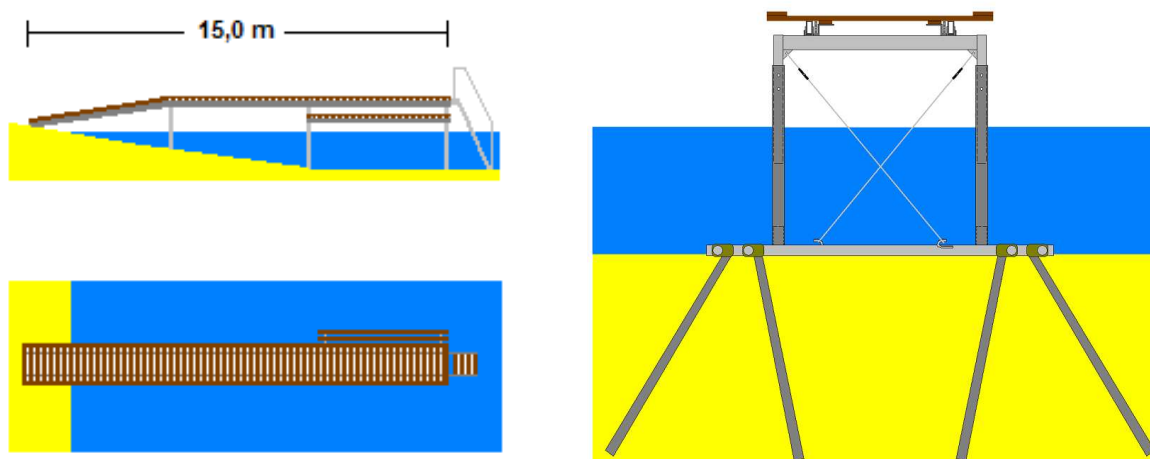
Figur 5: Skematisk tegning af broen (venstre billed) og dens forankring (højre billed)
